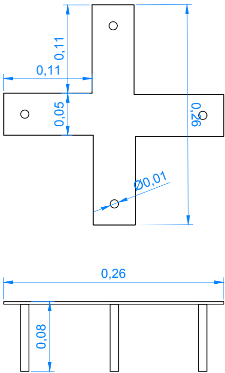
Grapa metálica en chapa de 3 mm y dos barillas de 10 mm que se insertan en los bastidores
