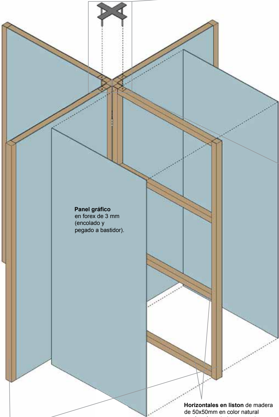
Verticales en liston de madera de 60x50mm en color natural con barniz mate transparente
