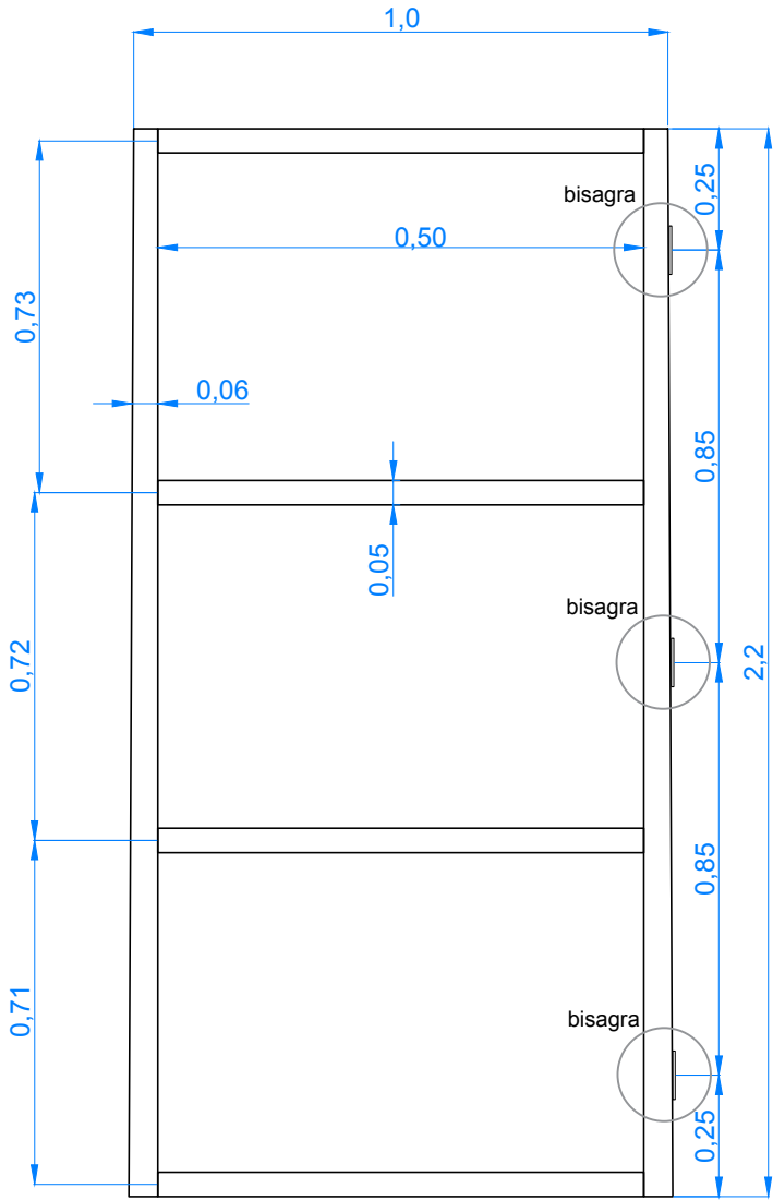
ALZADO ESTRUCTURA BASTIDOR
